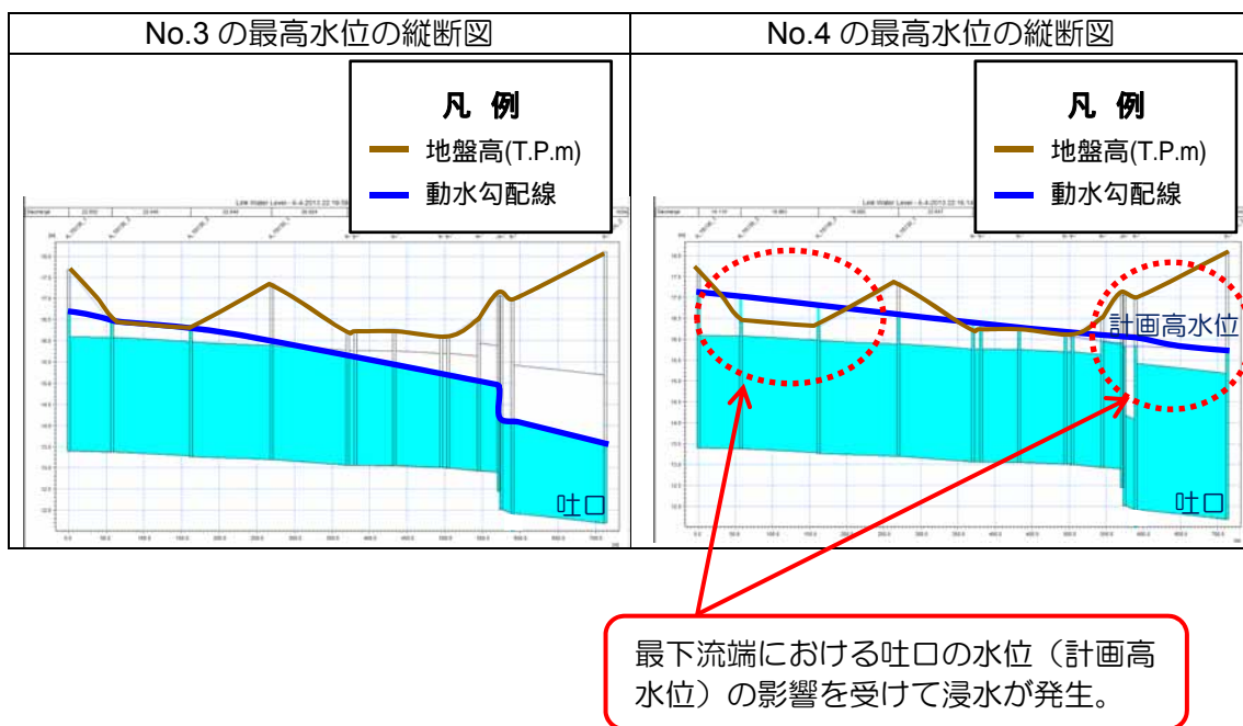
図 5.9 No.3 と No.4 の浸水箇所及び縦断図の比較
