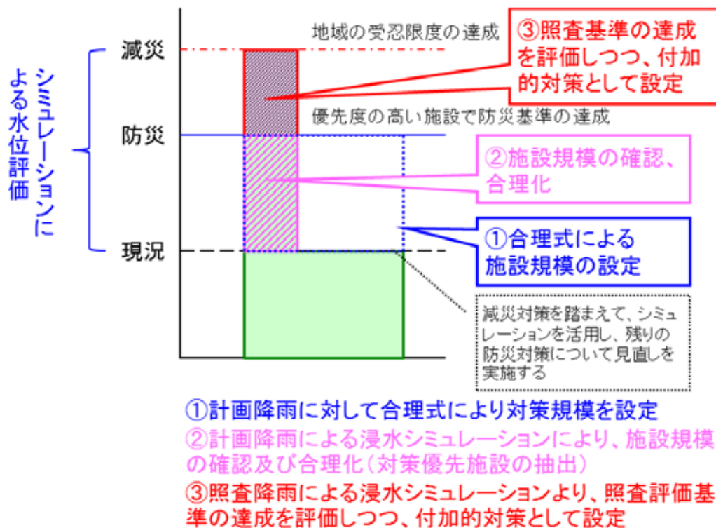
図 6.2 下水道事業における局地的ハード対策施設の規模設定の考え方
