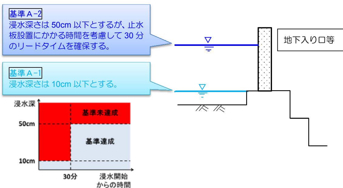
図 4.2 カテゴリーAにおける自助を組み合わせた評価基準達成のイメージ図
