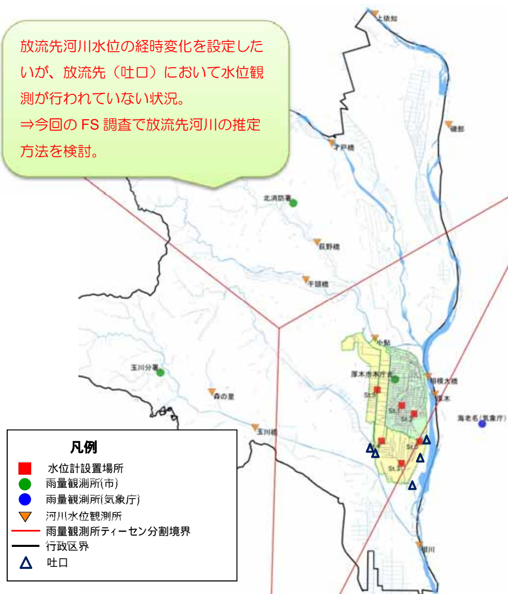
図 2.18 河川水位等観測地点の位置図
