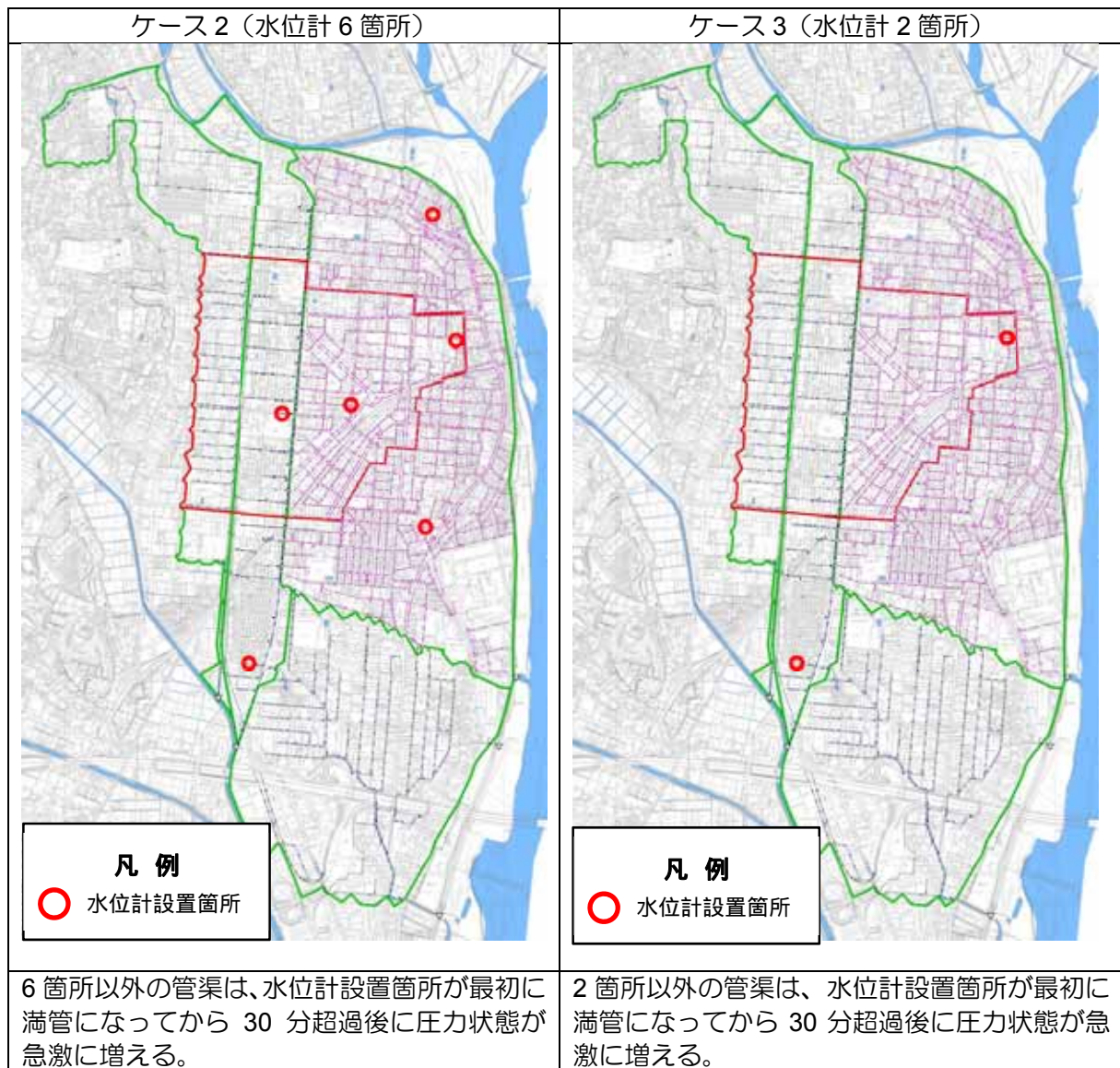
図 6.4 ケース別の水位計設置箇所（30分以内に圧力状態となる箇所）
