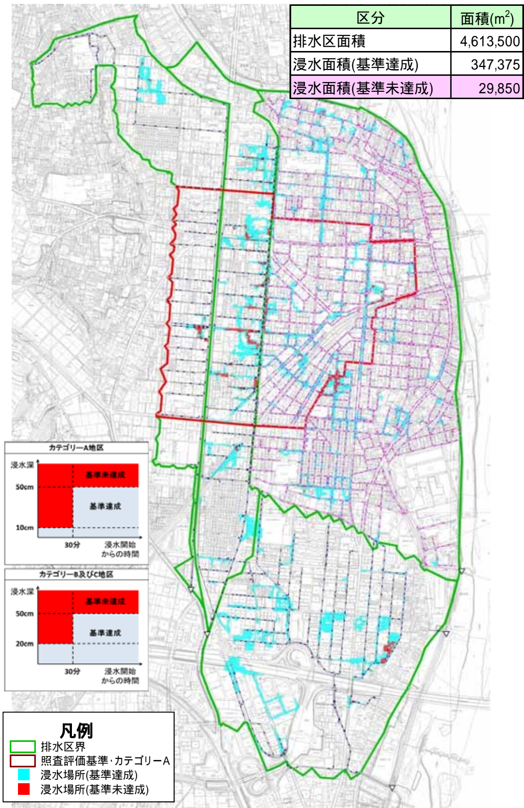
図 5.3 現況施設における照査基準達成状況（L 1' 降雨：2007/7/29 降雨）
