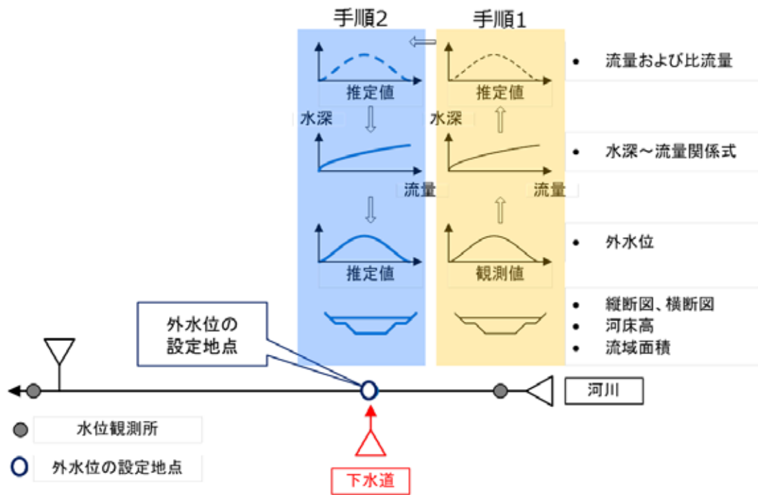
図 2.19 外水位推定方法の模式図
