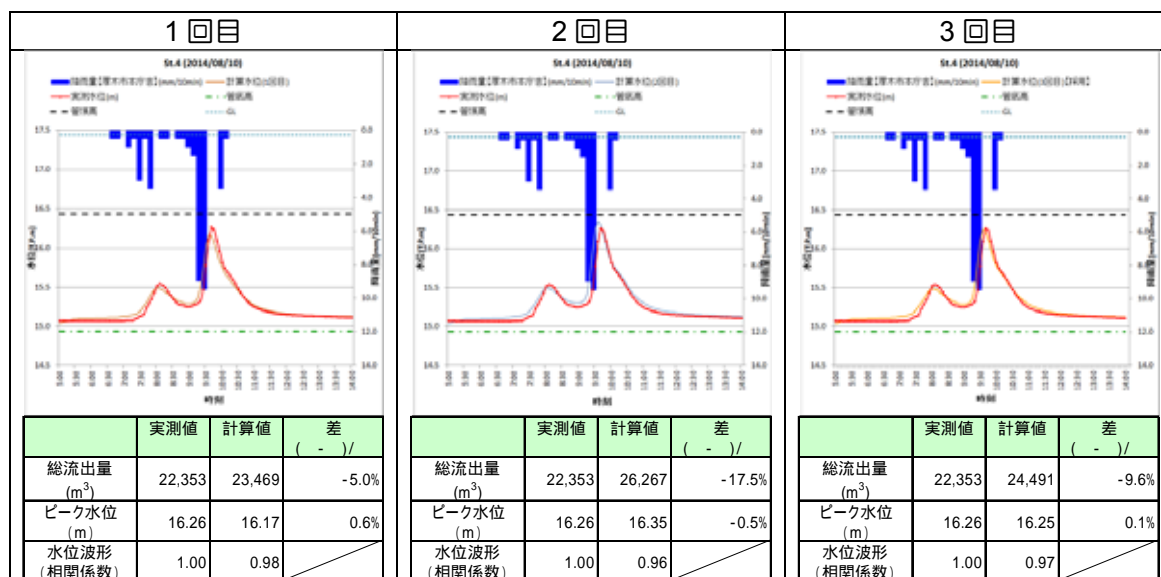
図 3.2 St.4 地点の各回キャリブレーション結果の例
