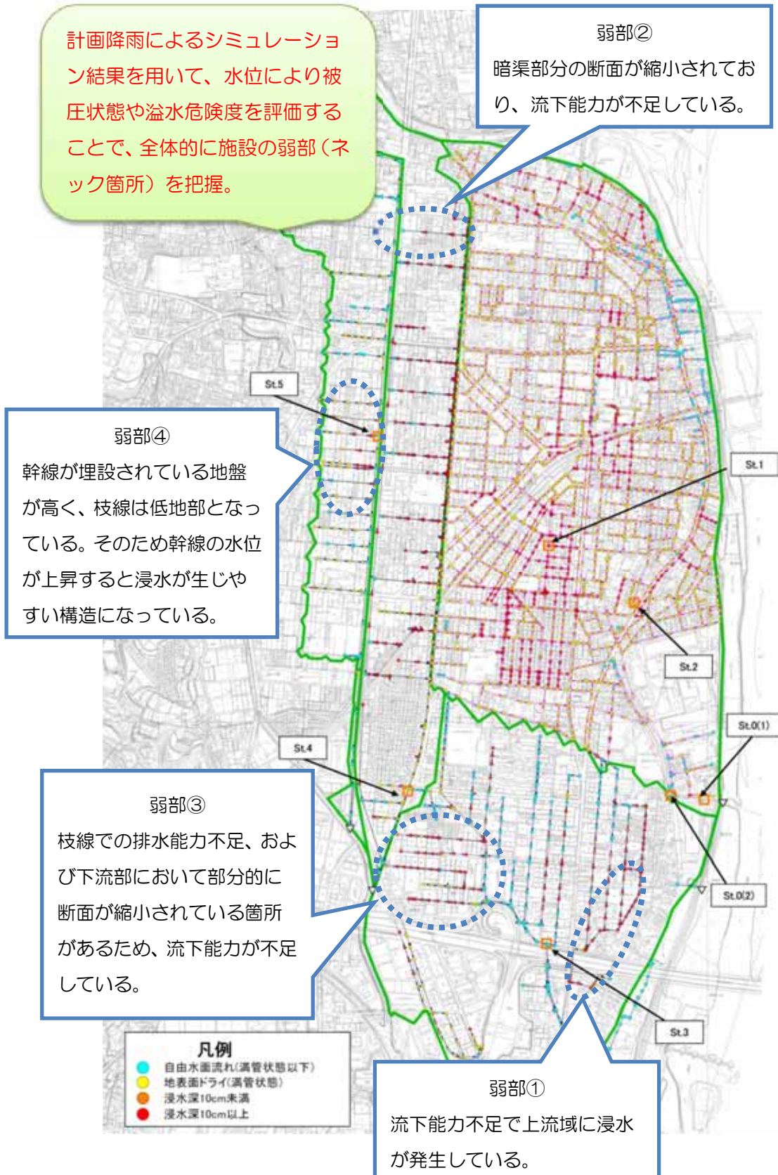
図 3.5 流出解析モデルによる計画降雨に対する現況施設の能力評価
