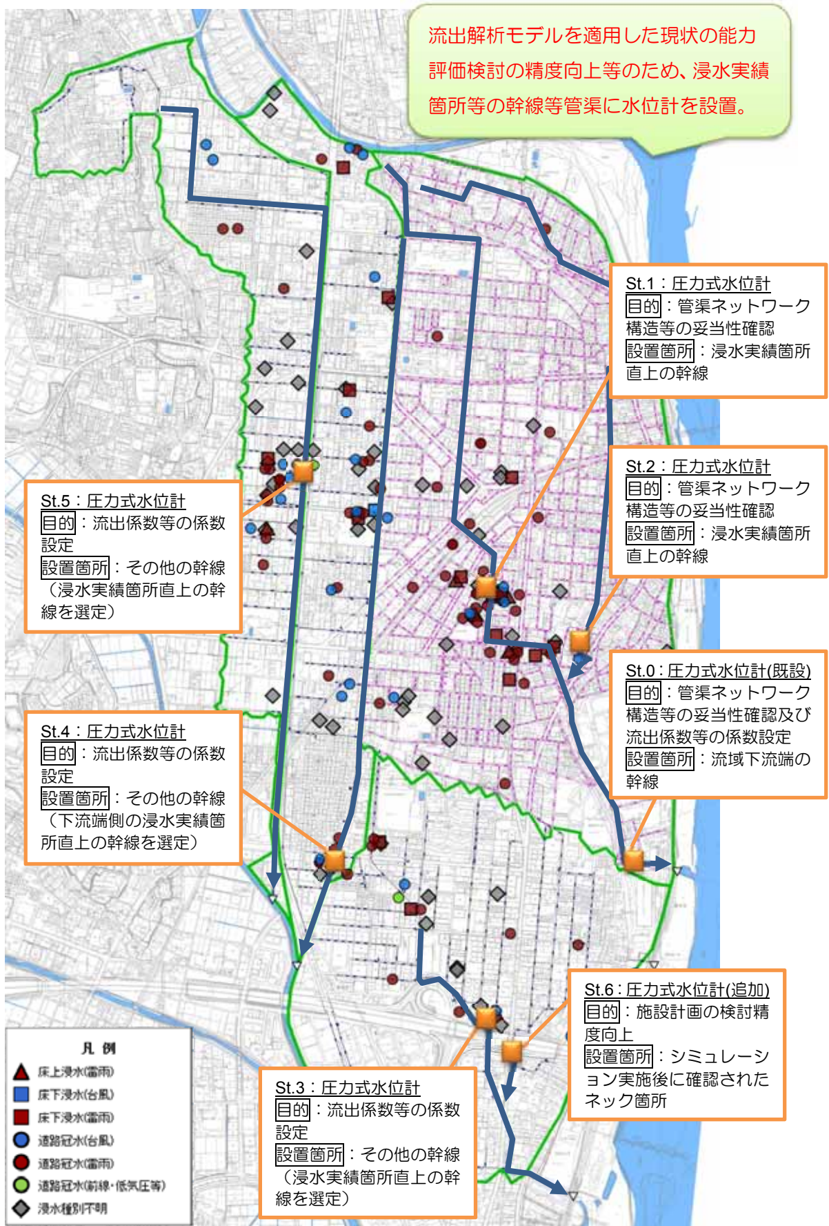
図 2.16 水位計設置位置
