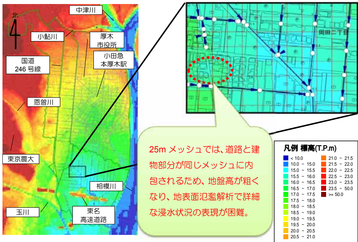
図 2.7 標高 25m メッシュの平面分布図
