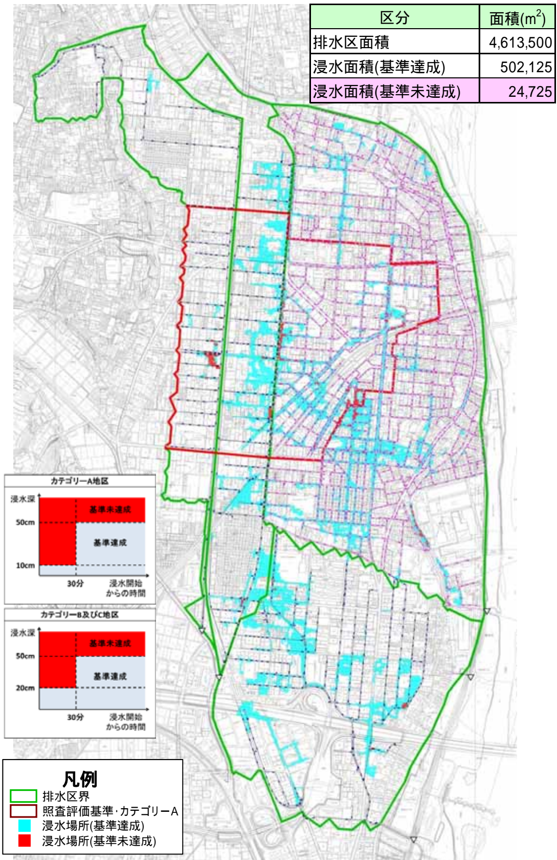
図 5.5 現況降雨における調査基準達成状況（L1' 降雨：2013/4/6 降雨，計画高水位）
