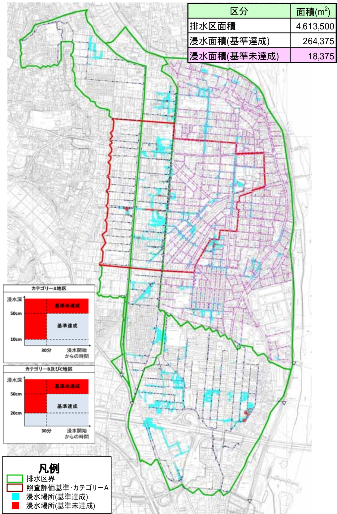
図 5.2 現況施設における照査基準達成状況 (L 1 降雨：計画降雨 51mm/hr)
