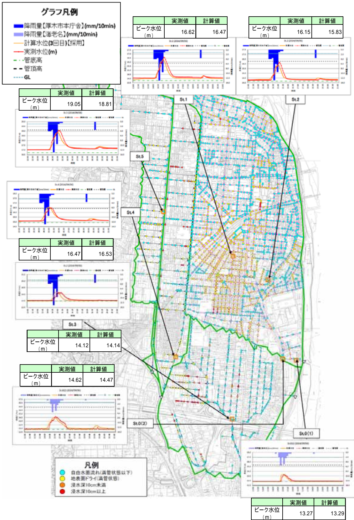
図 3.4 キャリブレーション結果 (3回目) の例 (2014/09/06 降雨)
