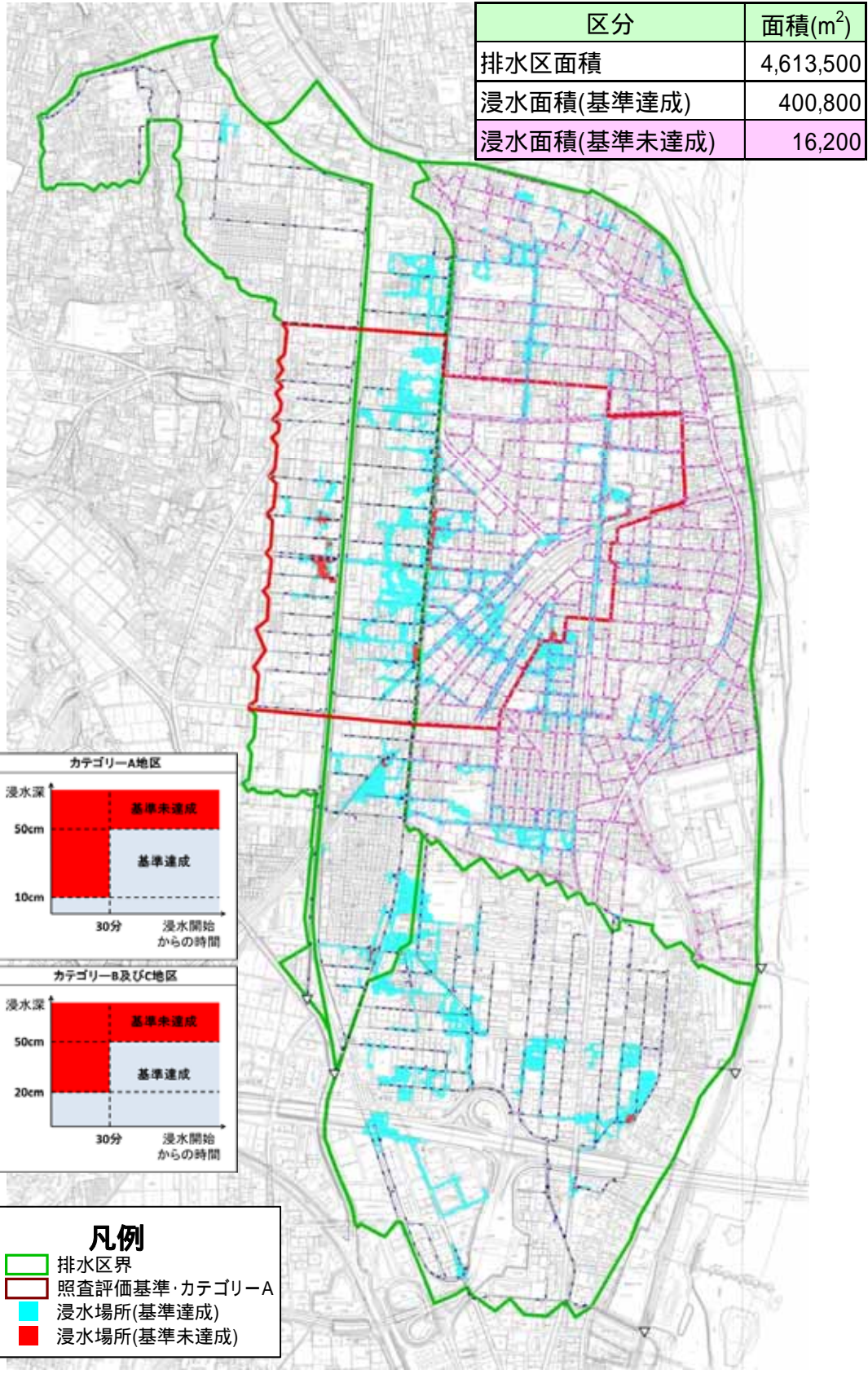
図 5.4 現況降雨における照査基準達成状況 (L 1' 降雨: 2013/4/6 降雨)
