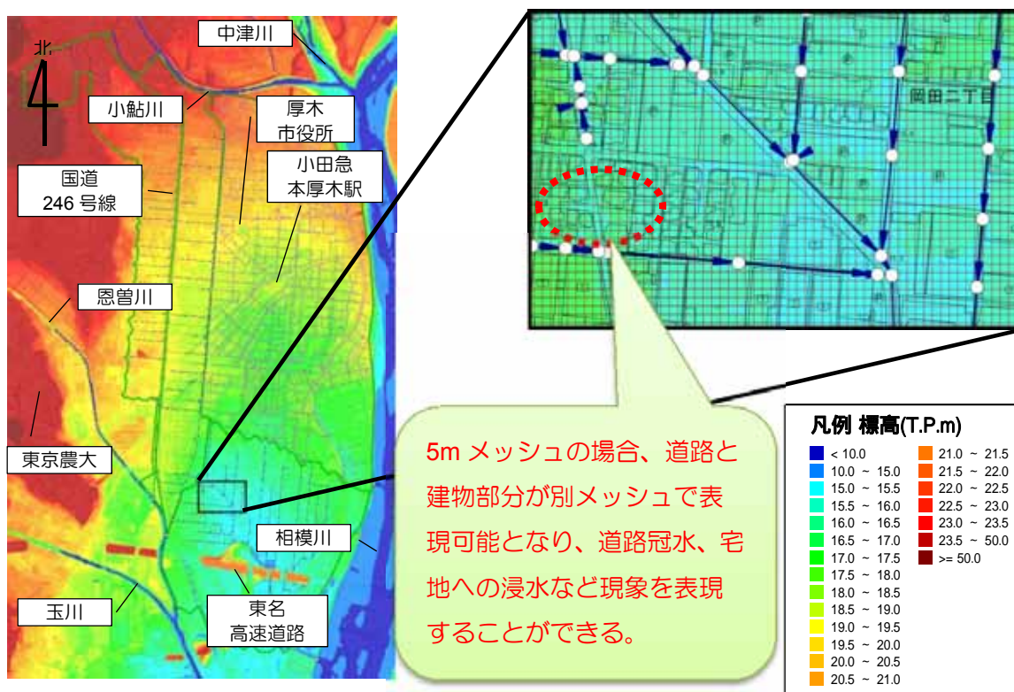
図 2.6 標高5mメッシュの平面分布図
