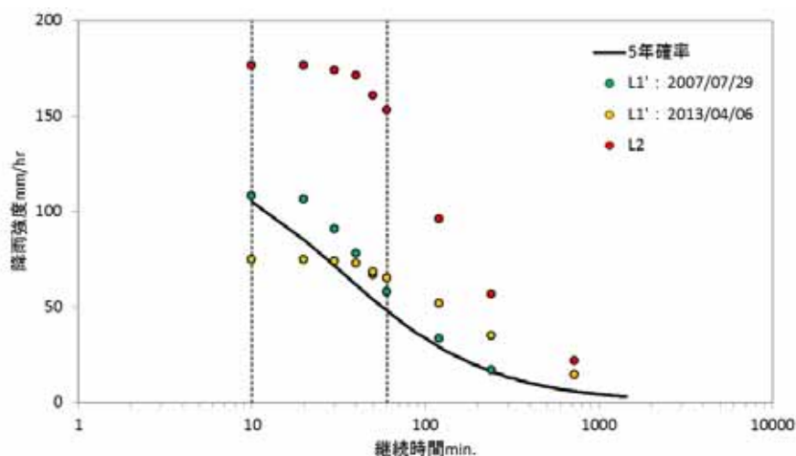
図 4.8 照査降雨の降雨ハイトグラフの設定結果
