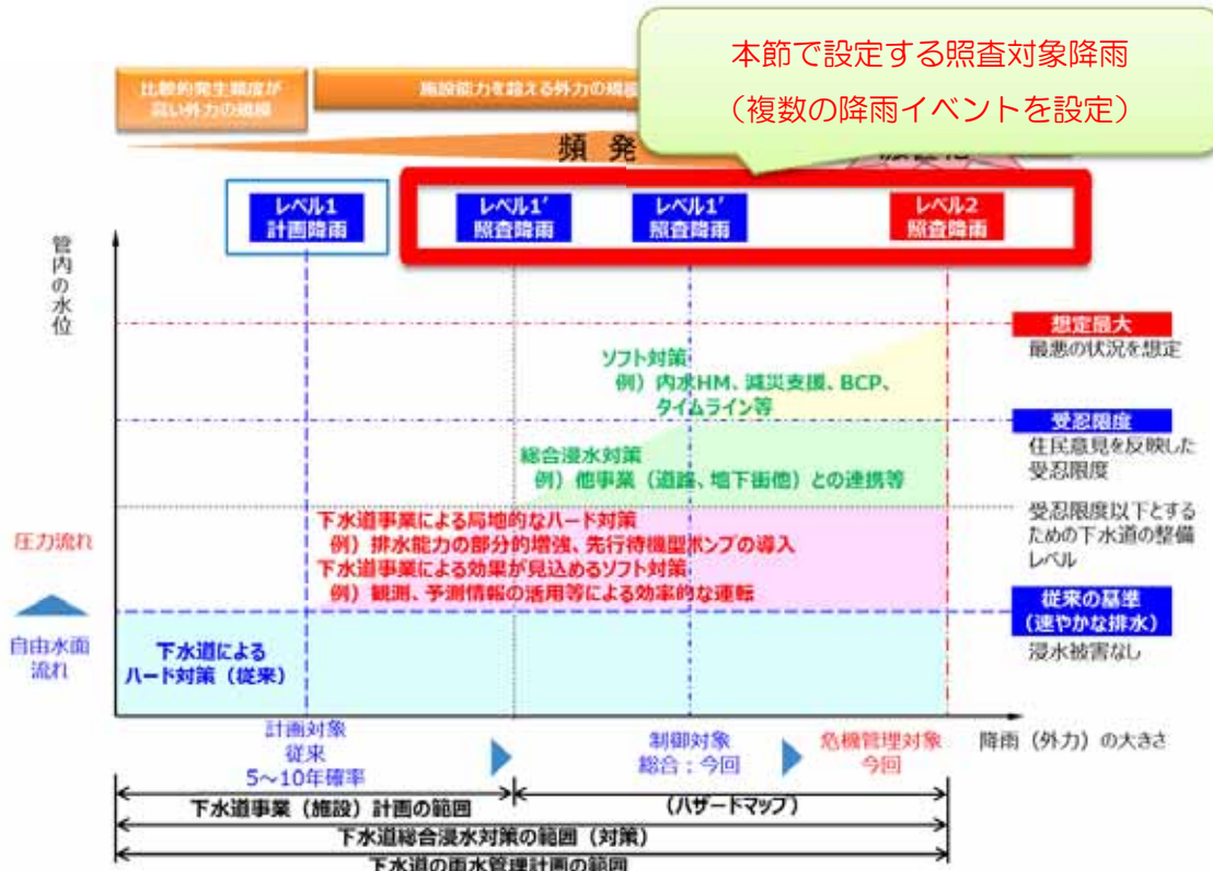
図 4.4 照査対象降雨の位置づけ
