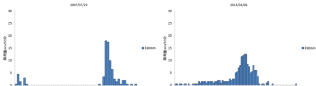
図 4.6 照査対象降雨 (L1') のハイトグラフ 21)
