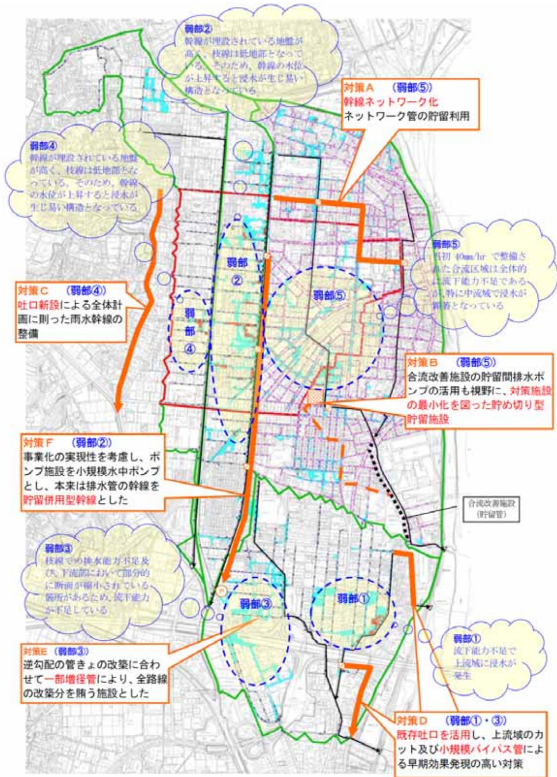
図 6.1 厚木市におけるハード対策施設（案）
