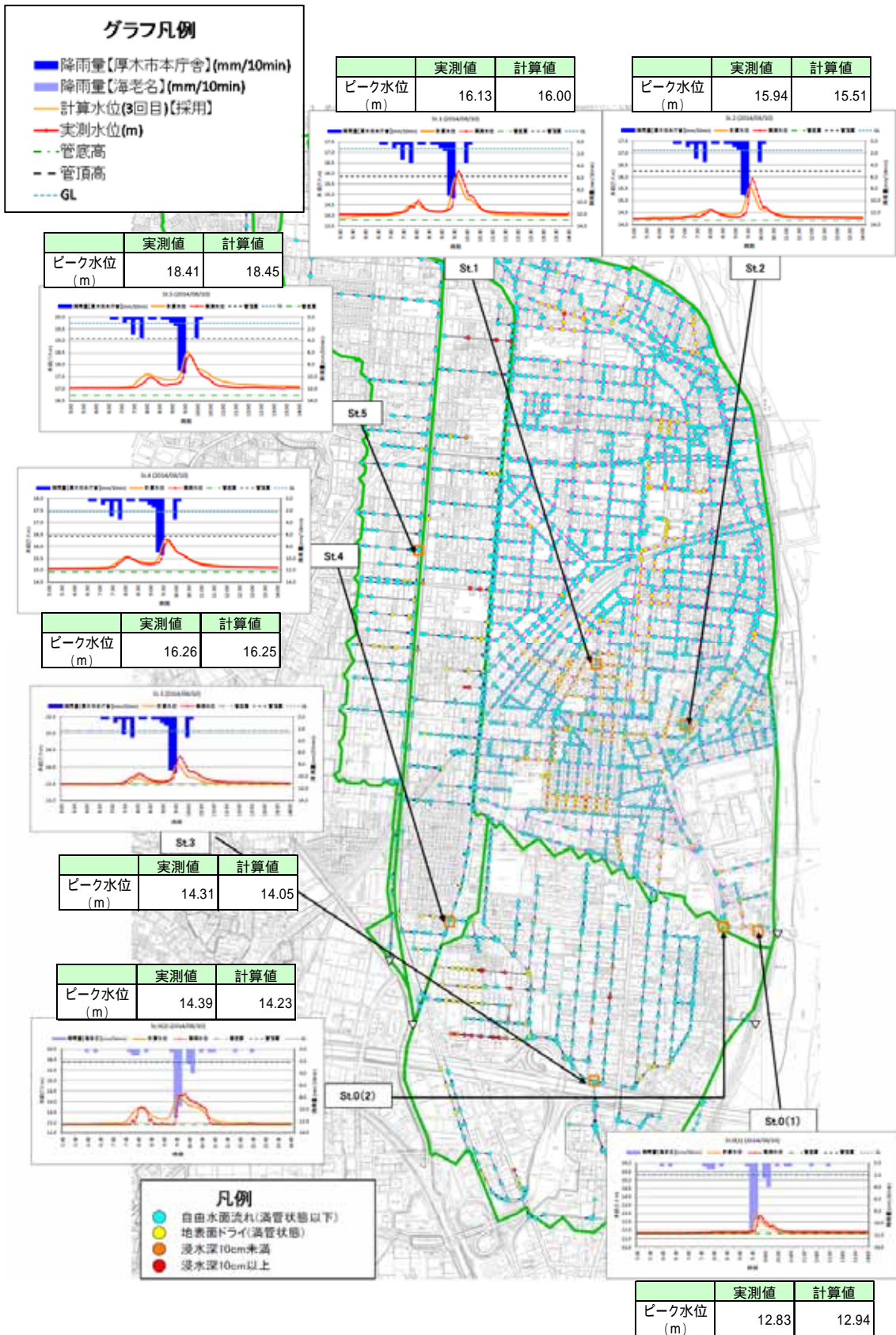
図 3.3 キャリブレーション結果 (3回目) の例 (2014/08/10 降雨)
