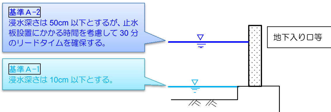
図 6.3 カテゴリーAにおける自助を組み合わせた評価基準達成のイメージ図(再掲)
