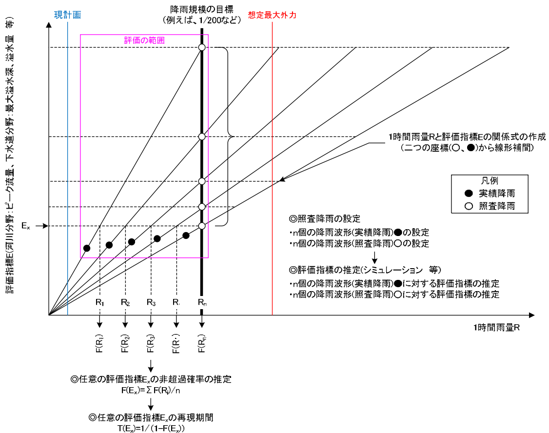
総合確率法の概念図
