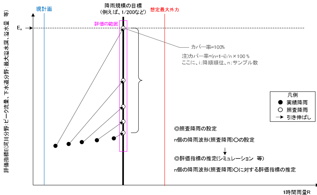
カバー率を用いる方法の概念図
