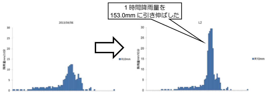
図 4.7 照査対象降雨（L2）のハイトグラフ
