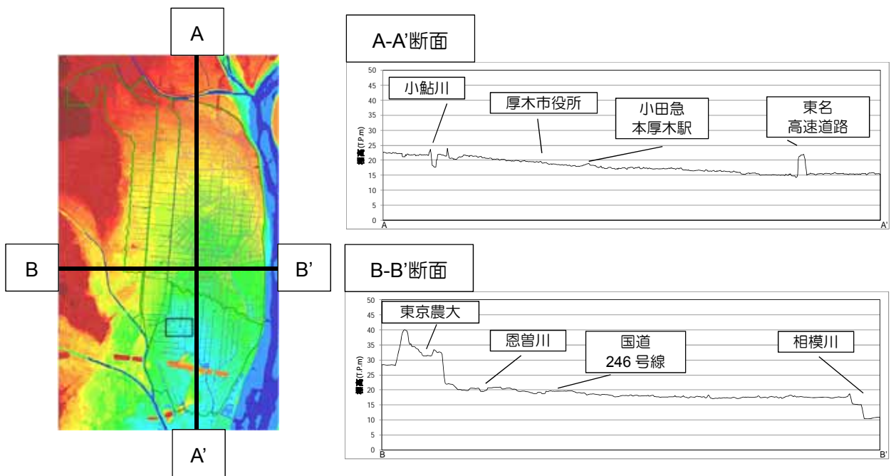
図 2.8 標高 5m メッシュの標高縦断図
