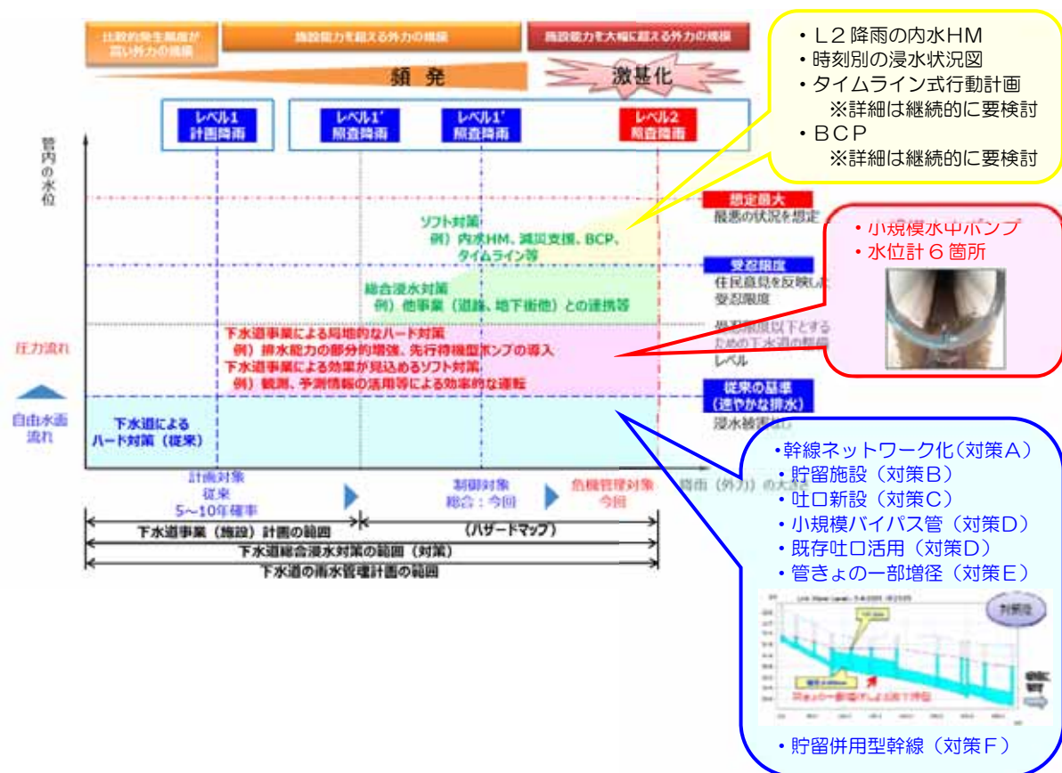
図 1.5 新たな考え方に基づく「雨水管理計画」の概念図と今回の対策内容の関係
