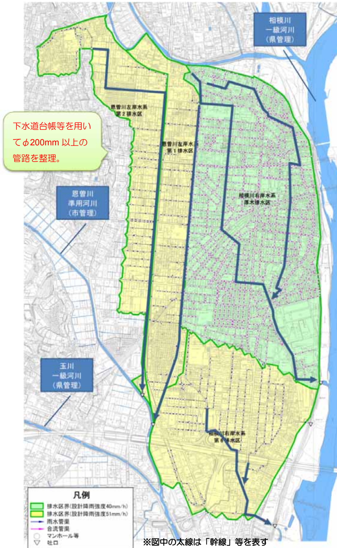
図 2.13 計画の対象範囲における管路網図
