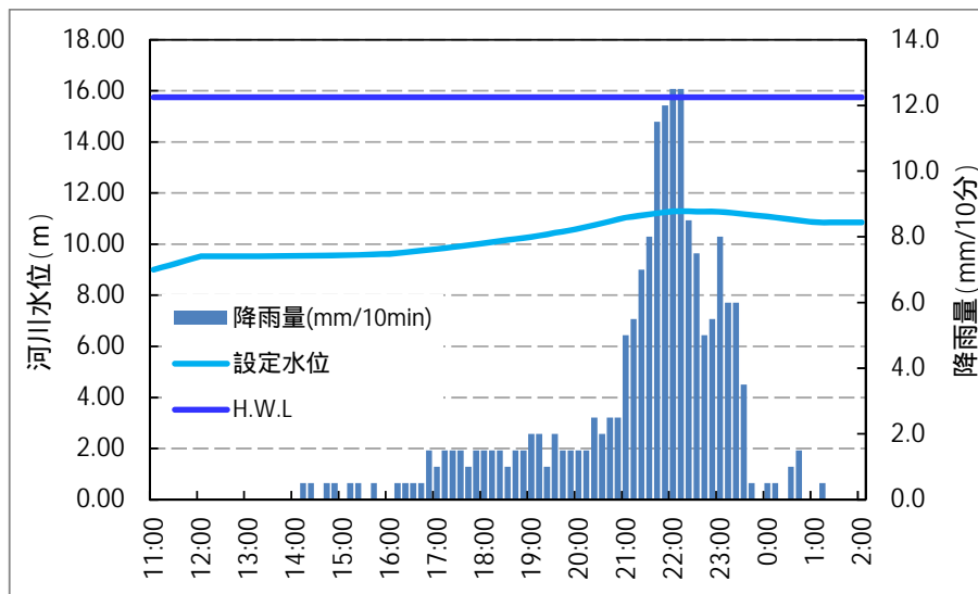
図 2.20 外水位設定例（2013/4/6 降雨：相模川①）
