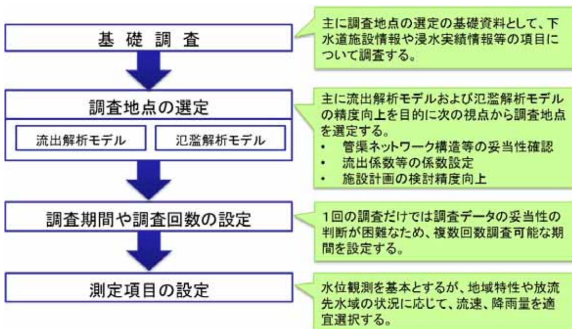
図 2.14 計画時における水位等観測の検討フロー（案）
