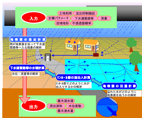
図 3.1 流出・氾濫解析モデルのイメージ
