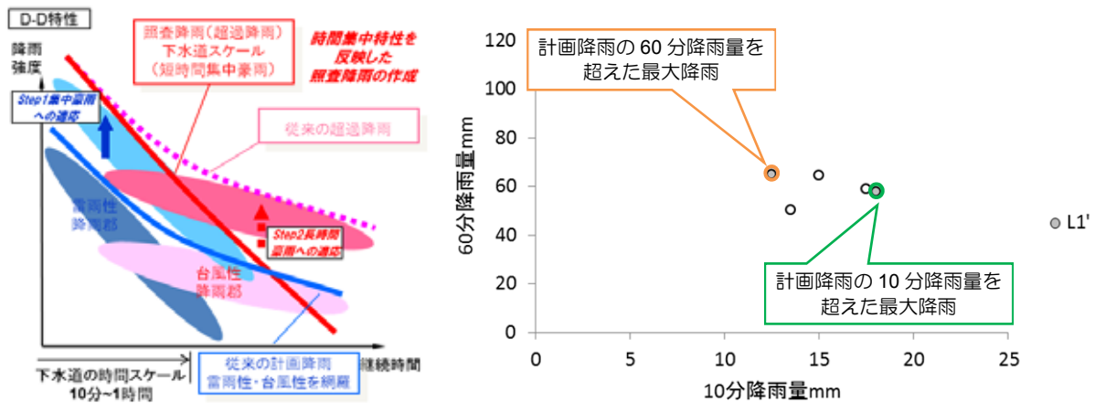
図 4.5 (左) DD 特性に着目した降雨イベントの抽出概念と(右) L1'降雨の特性
